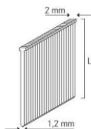
KMR Mini-brads 18GA Durchmesser 1,2 mm Länge 15 - 55 mm
